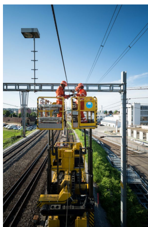
Source: Suva liste de contrôle réf. 67064/2: «Plateformes élévatrices»
