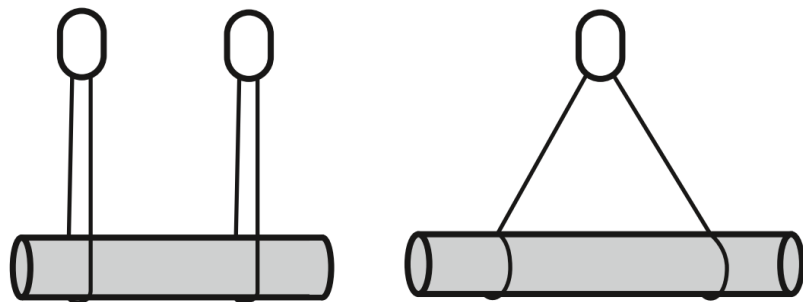
Source: Suva liste de contrôle réf. 67017: «Élingues»
